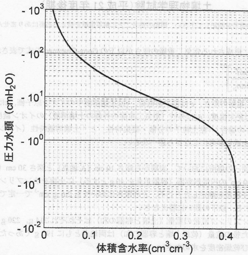
図1 土壤水分特性曲線
