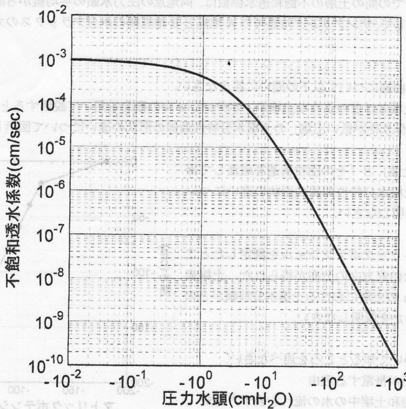
図2 不飽和透水係数と圧力水頭の関係
